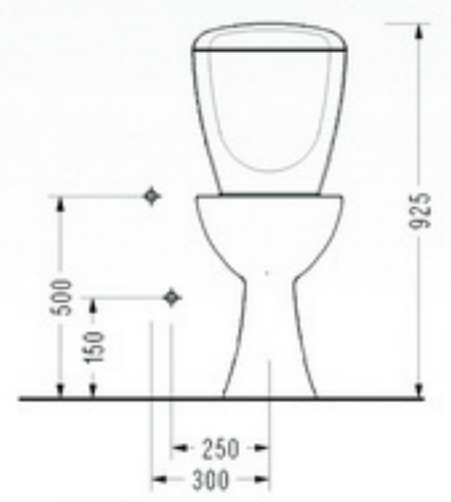
• 7645 Klozet (alttan çıkışlı) • 7648 Rezervuar
