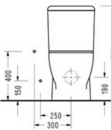
• SM02 BTW Takım Klozeti • SM04 Rezervuar
