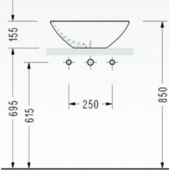
• 2012 Çanak Lavabo Sadece kumandasız bataryalar ile kullanılır.
