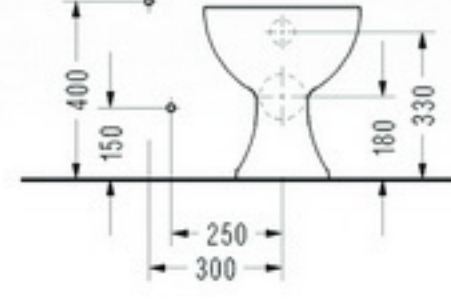
• 0902 Arkadan Çıkışlı Klozet
