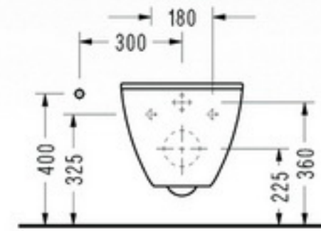
• SM10 Asma Klozet
