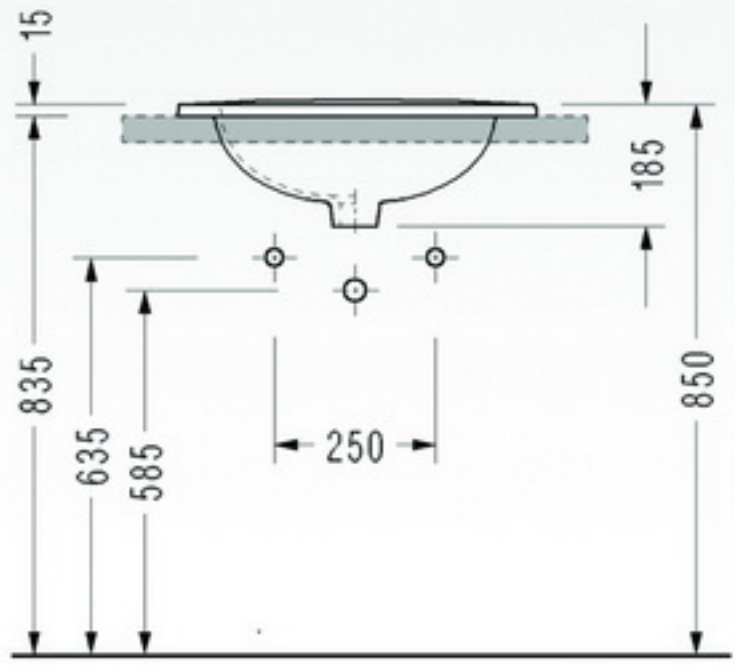
• 1841 Lavabo (tezgaha gömülü)
