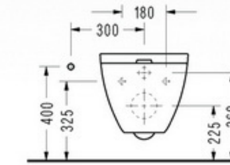
• SM13 Asma Klozet
