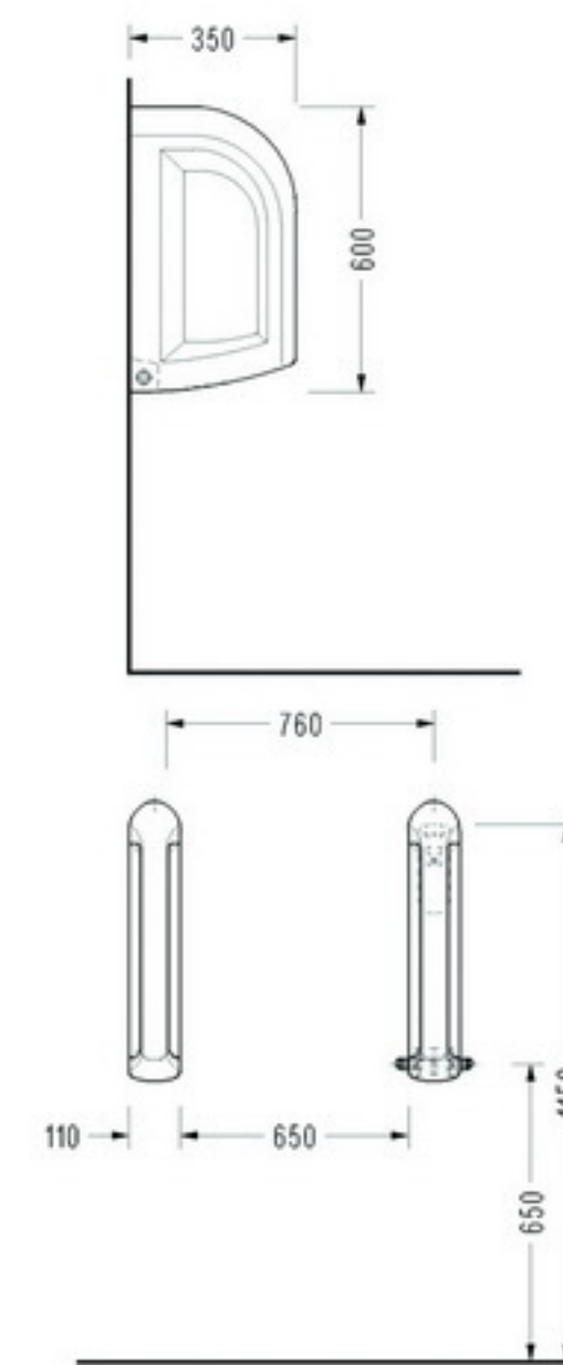
• 6807 Pisuar Ara Bölme
