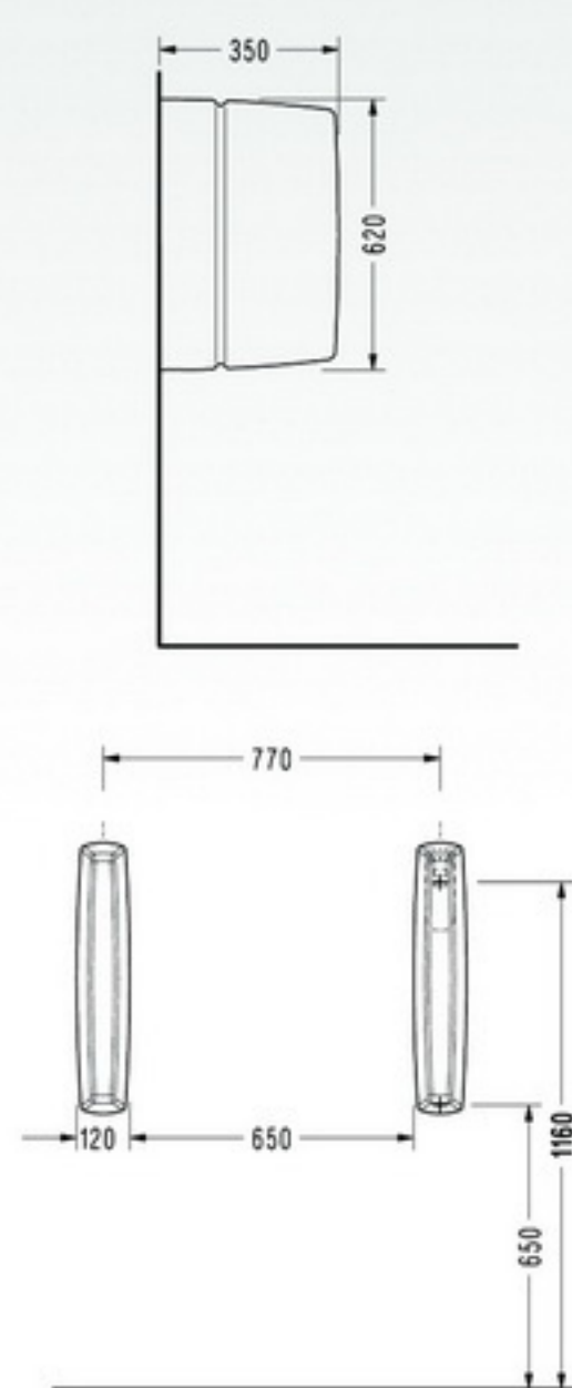
• DG20 Pisuar Ara Bölmesi
