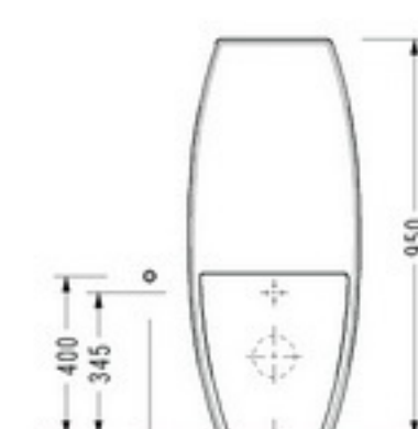
• 8911 BTW Standart Klozet • 8949 Monoblok Rezervuar
