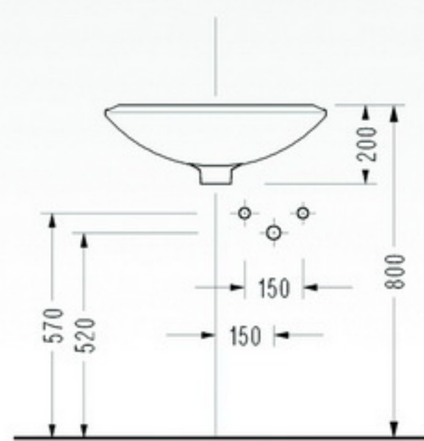
• 0433 Köşe Lavabo 150400300166 - Havluluk barı opsiyoneldir.
