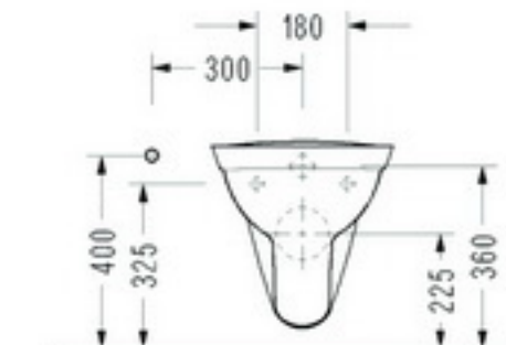
• O422 Asma Klozet
