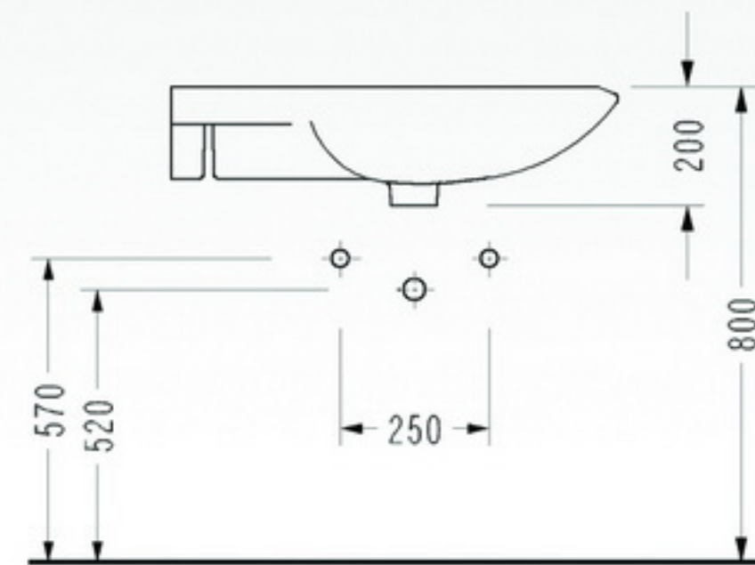
• 0435 Soldan Etajerli Lavabo 150400300167 - Havluluk barı opsiyoneldir.
