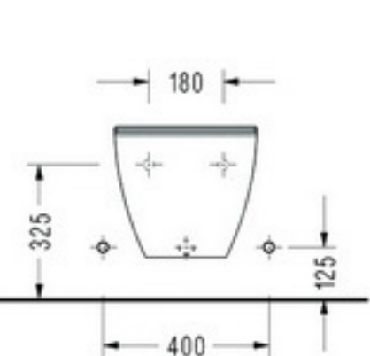
• SM19 Asma Bide
