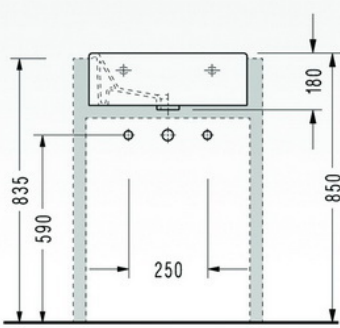
• 2043 Lavabo (yarım tezgah üstü)
