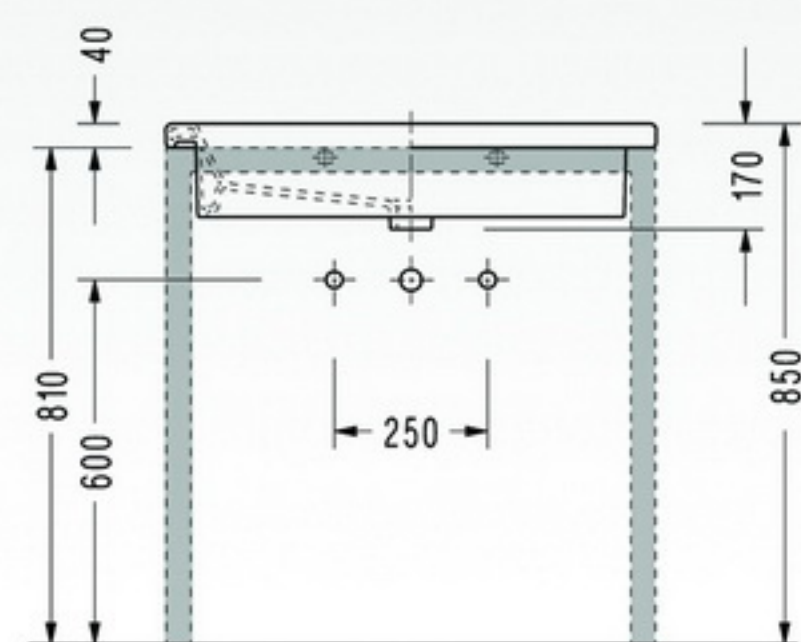
• 8931 Lavabo (tezgaha gömülü)
