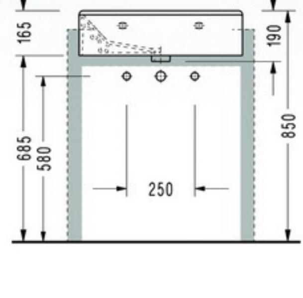
• 2044 Dikdörtgen Lavabo (yarım tezgah üstü)
