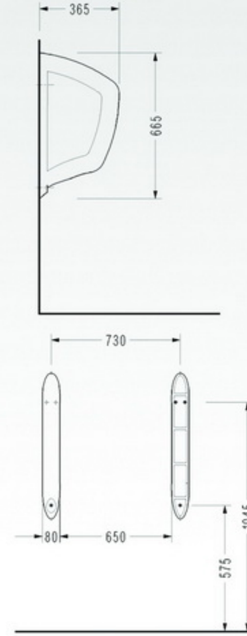
• 0140 Pisuar Ara Bölmesi
