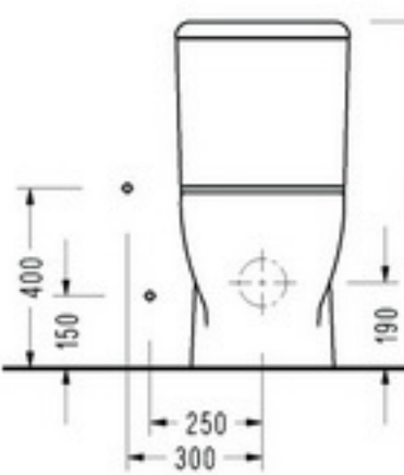
• SM16 Universal BTW Klozet • SM04 Rezervuar
