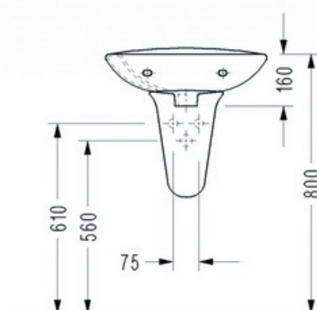
• 2841 Lavabo • 2822 Yarım Ayak
