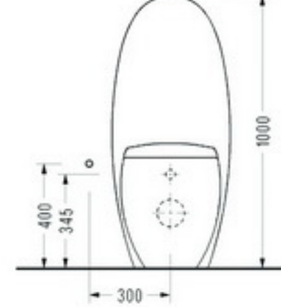
• 7411 BTW Standart Klozet • 7446 Monoblok Rezervuar
