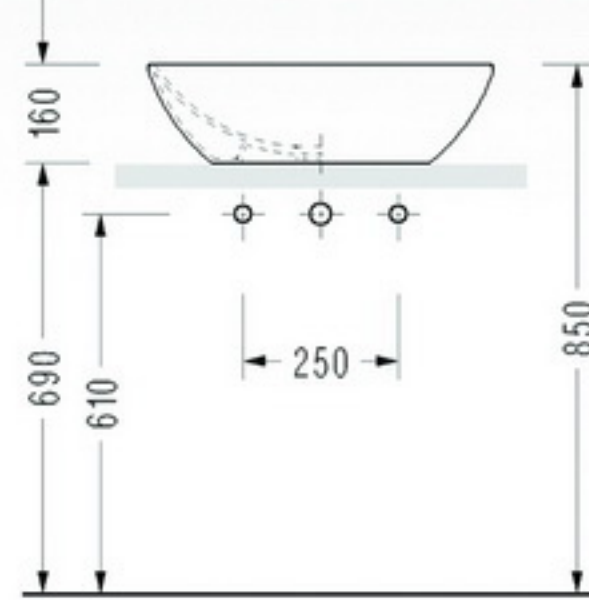
• CH33 Çanak Lavabo Sadece kumandasız bataryalar ile kullanılır.
