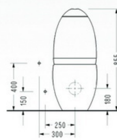
• 7402 BTW Takım Klozeti • 7404 Rezervuar
