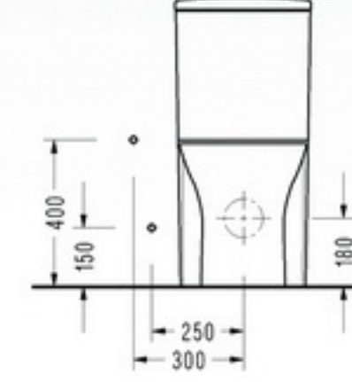
• DP02 BTW Takım Klozeti • 6748 Rezervuar
