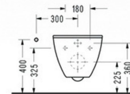
• SM10 Asma Klozet
