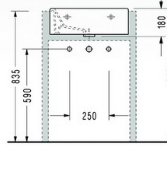
• 2043 Kare Lavabo (yarım tezgah üstü)
