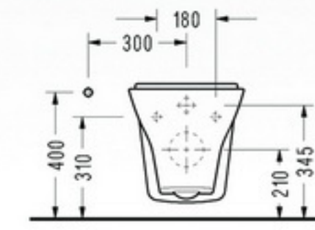
• DP10 Asma Klozet
