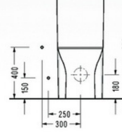
• DP02 BTW Takım Klozeti • AD29 Rezervuar
