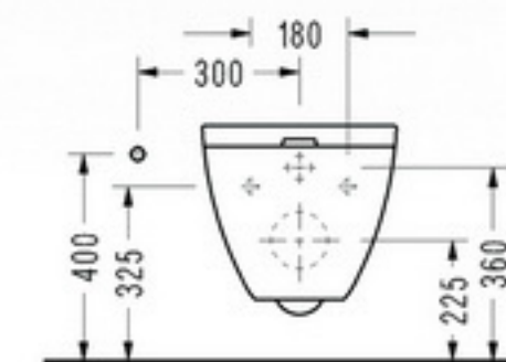
• SM13 Asma Klozet
