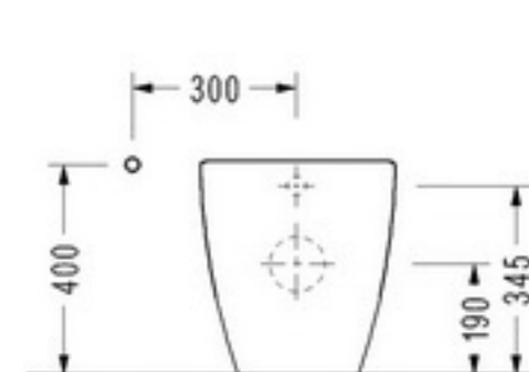
• 8911 BTW Standart Klozet
