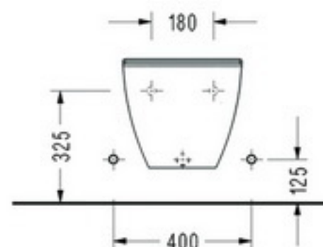
• SM19 Asma Bide
