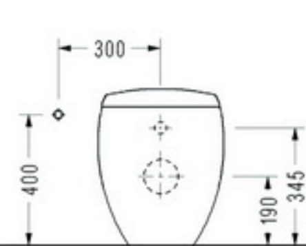
• 7411 BTW Standart Klozet
