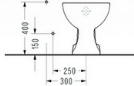
• 0602 Altan Çıkışlı Klozet
