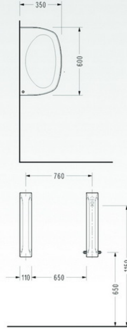
• 0120 Pisuar Ara Bölmesi
