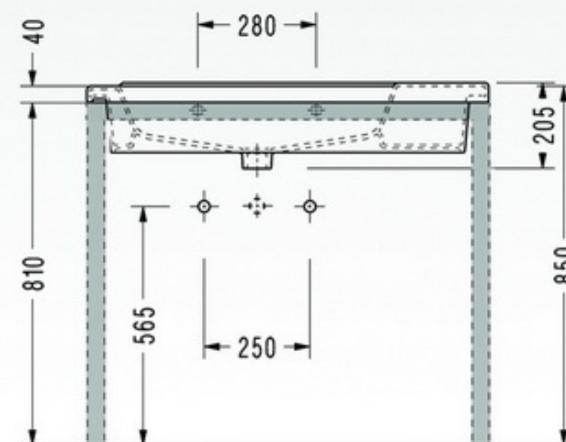
• 8934 Lavabo (tezgaha gömülü)
