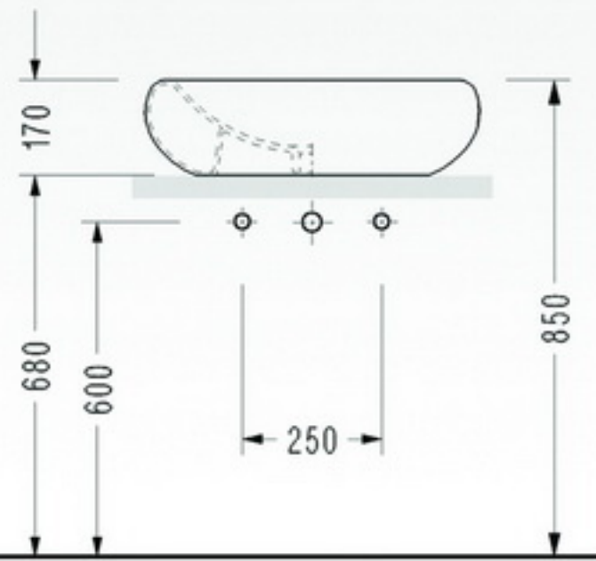
• 7433 Lavabo (tezgah üstü)
