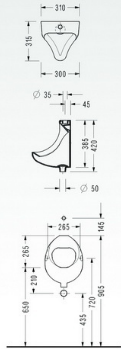
• 0149UZ Pisuar (üstten temiz su çıkışlı)
