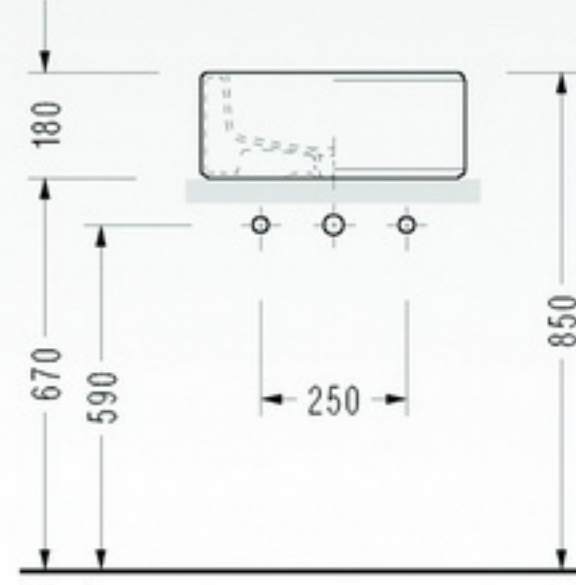
• 2052 Silindirik Lavabo Sadece kumandasız bataryalar ile kullanılır.
