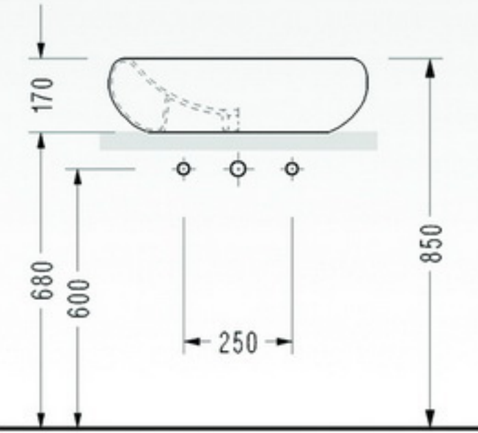
• 7425 Lavabo (tezgah üstü)
