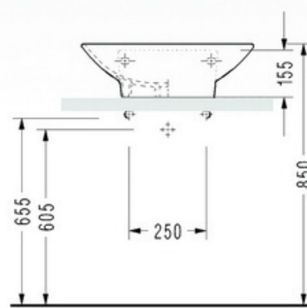
• CH01 Çanak Lavabo
