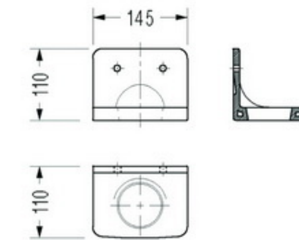
• FU20 Seramik Bardaklık
