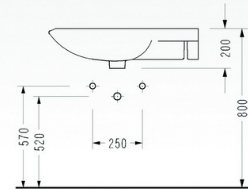
• 0434 Sağdan Etajerli Lavabo 150400300167 - Havluluk barı opsiyoneldir.
