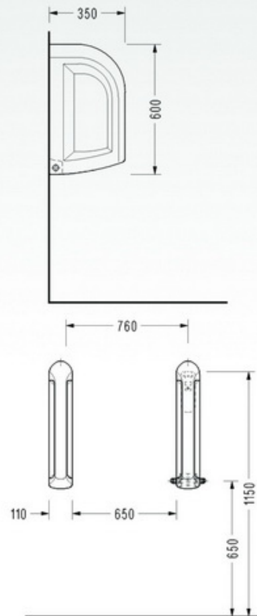
• 6807 Pisuar Ara Bölmesi
