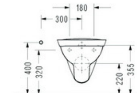
• O412 Asma Klozet
