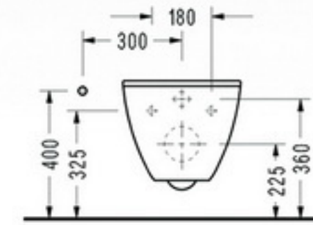
• SM15 Asma Klozet
