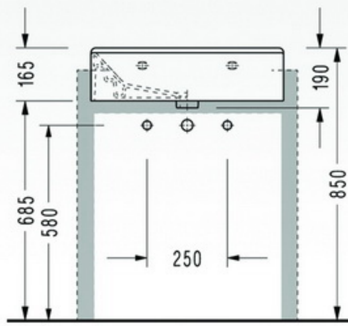
• 2044 Lavabo (yarım tezgah üstü)
